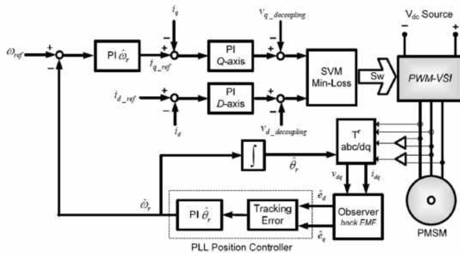
Rys. 2. Bezczyjnikowy układ sterowania połowo-zorientowanego silnikiem PMSM z wykorzystaniem estymatora PLL [6]
