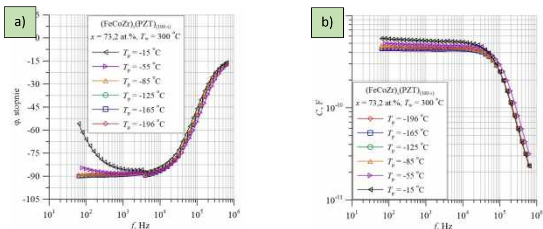
Rysunek 2. Zależności częstotliwościowe: a) kąta przesunięcia fazowego oraz b) pojemności nanokompozytu (FeCoZr) x (PbZrTiO 3 ) 100-x poddanego obróbce termicznej w temperaturze T_w = 300^\circ\text{C}
